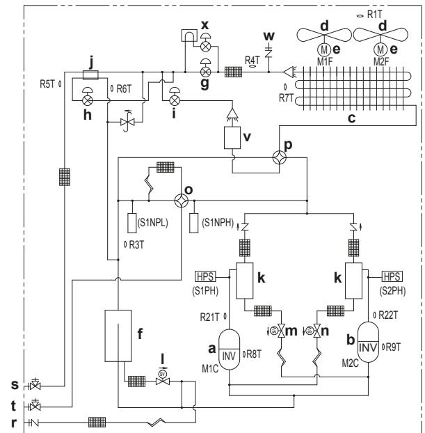
Схема трубопроводов: RYYQ14~20
