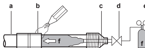
a Трубопровод хладагента b Детали, подвергаемые пайке c Изолирующая обмотка d Ручной клапан e Редукционный клапан f Азот
